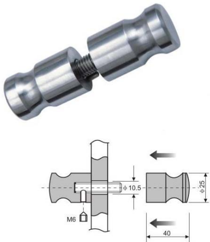
Door Knob/ REF:: 600007
