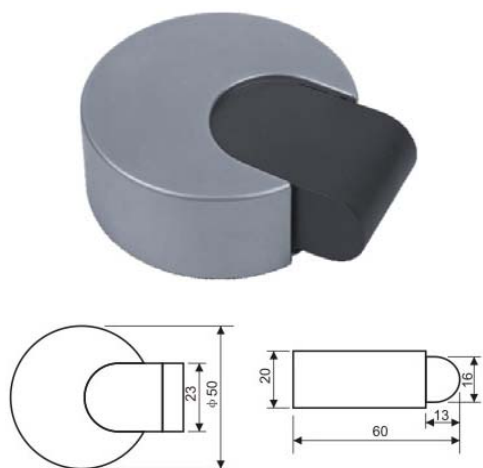
Door Stopper/ REF:: 500041
