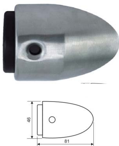
Door Stopper/ REF:: 500059
