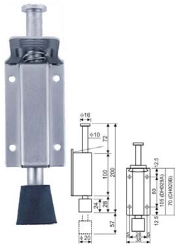
Door Holder/ REF:: 500029
