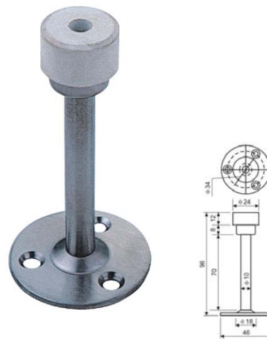
Door Stopper/ REF:: 500023
