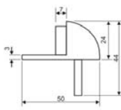
Door Stopper/ REF:: 500002
