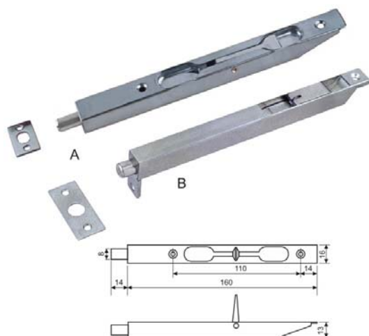
Door Bolt/ REF:: 510103 & 510203
